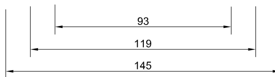
Griff Ansicht Oben 1:2
